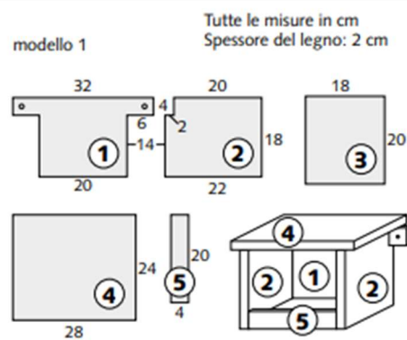
Esempio di cassetta nido (A. Persico) e istruzioni per la costruzione (BirdLife)
